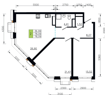
План 22-23 этажа Корпус 1 Секция 3 квартира №4
