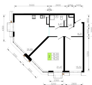
План 11-16 этажа Корпус 1 Секция 3 квартира №4
