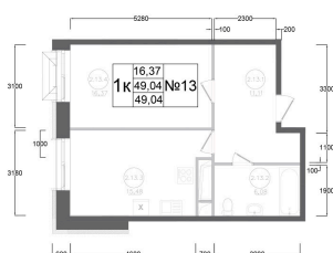
План типового 4-11 этажа Корпус 1 Секция 2 Квартира №13
