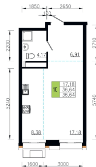
План 11-16 этажа Корпус 1 Секция 3 квартира №3
