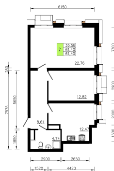
План 11-16 этажа Корпус 1 Секция 3 квартира №8
