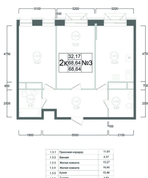
План типового 4-11 этажа Корпус 1 Секция 1 Квартира №3
