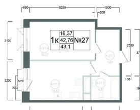
План 3 этажа Корпус 1 Секция 4 Квартира №27
