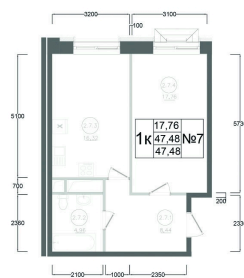
План типового 12-15 этажа Корпус 1 Секция 2 Квартира №7
