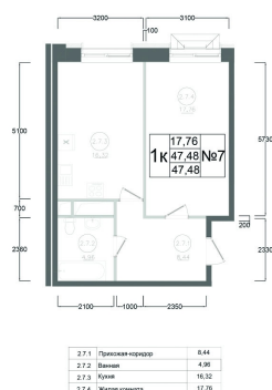
План типового 12-15 этажа Корпус 1 Секция 2 Квартира №7
