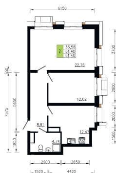
План 21 этажа Корпус 1 Секция 3 квартира №8
