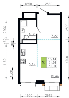
План 3-9 этажа Корпус 1 Секция 1 квартира №3
