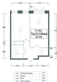
План 2 этажа Корпус 1 Секция 1 Квартира №4
