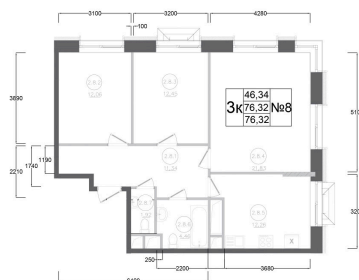
План 16 этажа Корпус 1 Секция 2 Квартира №8
