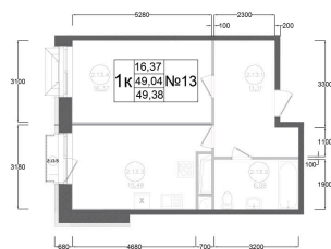
План 3 этажа Корпус 1 Секция 2 Квартира №13
