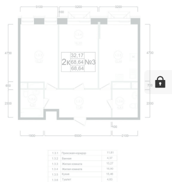
План типового 4-11 этажа Корпус 1 Секция 1 Квартира №3
