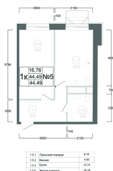
План 2 этажа Корпус 1 Секция 1 Квартира №5
