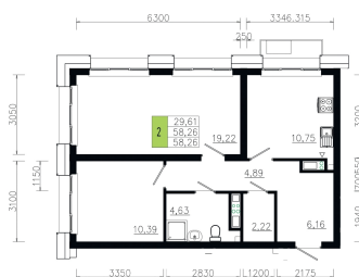
План типового этажа Корпус 2 квартира №6
