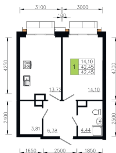
План 3-9 этажа Корпус 1 Секция 3 квартира №7
