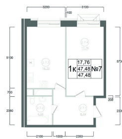
План 2 этажа Корпус 1 Секция 2 Квартира №7
