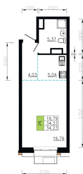
План 17 этажа Корпус 1 Секция 2 квартира №2
