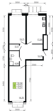
План 2 этажа Корпус 1 Секция 2 квартира №5
