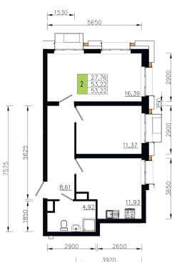
План 3-9 этажа Корпус 1 Секция 3 квартира №8
