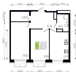
План 3-9 этажа Корпус 1 Секция 2 квартира №4
