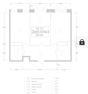
План типового 4-11 этажа Корпус 1 Секция 1 Квартира №3
