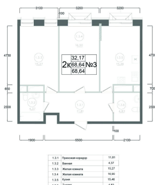
План типового 12-15 этажа Корпус 1 Секция 1 Квартира №3
