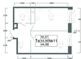
План типового 12-15 этажа Корпус 1 Секция 2 Квартира №11
