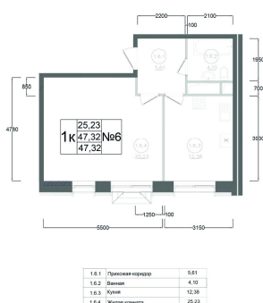
План типового 12-15 этажа Корпус 1 Секция 1 Квартира №6
