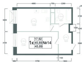
План 16 этажа Корпус 1 Секция 2 Квартира №14
