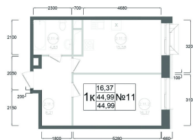
План типового 4-11 этажа Корпус 1 Секция 2 Квартира №11
