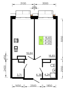
План 11-16 этажа Корпус 1 Секция 3 квартира №7
