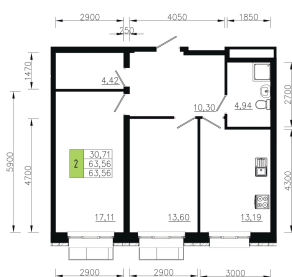
План 2 этажа Корпус 1 Секция 2 квартира №4
