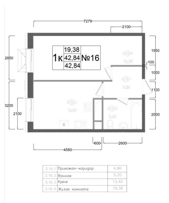
План типового 4-11 этажа Корпус 1 Секция 3 Квартира №16
