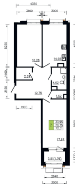
План 10 этажа Корпус 1 Секция 3 квартира №1
