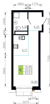
План 3-9 этажа Корпус 1 Секция 1 квартира №4
