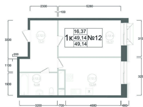
План 16 этажа Корпус 1 Секция 2 Квартира №12
