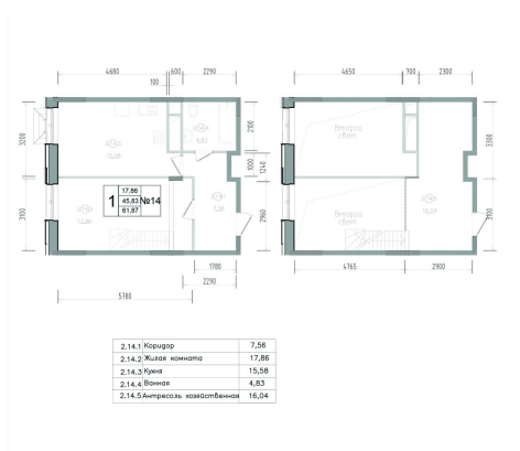
План 17 этажа Корпус 1 Секция 2 Квартира №14
