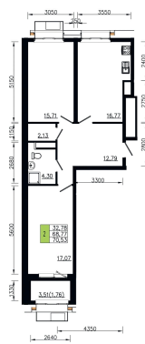
План 10 этажа Корпус 1 Секция 5 квартира №5
