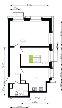
План 10 этажа Корпус 1 Секция 3 квартира №8
