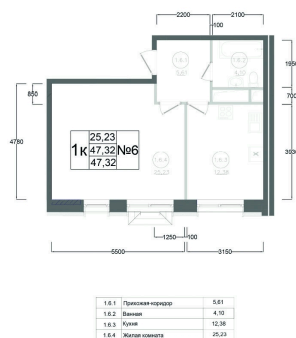
План типового 4-11 этажа Корпус 1 Секция 1 Квартира №6
