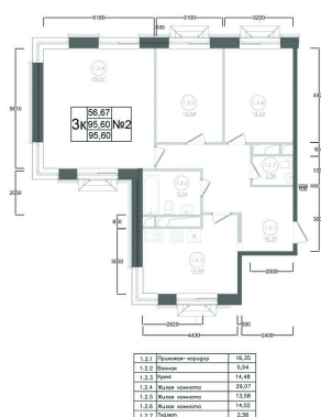
План типового 12-15 этажа Корпус 1 Секция 1 Квартира №2
