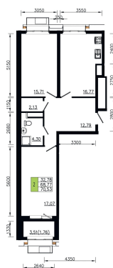
План 17 этажа Корпус 1 Секция 2 квартира №5
