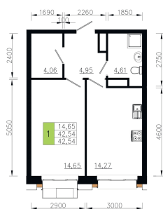
План 20 этажа Корпус 1 Секция 3 квартира №3
