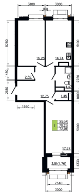
План 19 этажа Корпус 1 Секция 3 квартира №1
