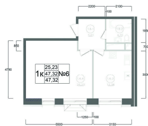
План типового 4-11 этажа Корпус 1 Секция 1 Квартира №6
