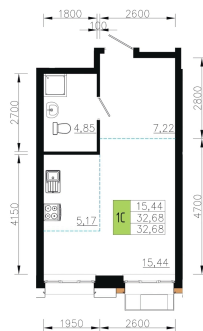
План 2 этажа Корпус 1 Секция 1 квартира №3
