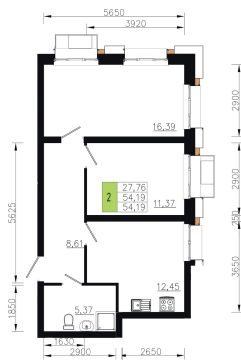
План 2 этажа Корпус 1 Секция 3 квартира №8
