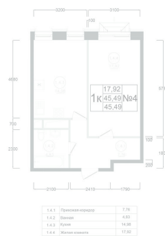
План типового 4-11 этажа Корпус 1 Секция 1 Квартира №4
