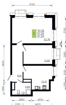
План 22-23 этажа Корпус 1 Секция 3 квартира №8
