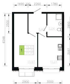
План 2 этажа Корпус 1 Секция 3 квартира №3
