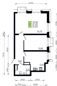
План 20 этажа Корпус 1 Секция 3 квартира №8
